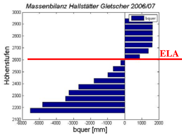
Abbildung 4.4c. Mittlere spezifische Massenbilanz der Höhenstufen und ELA
